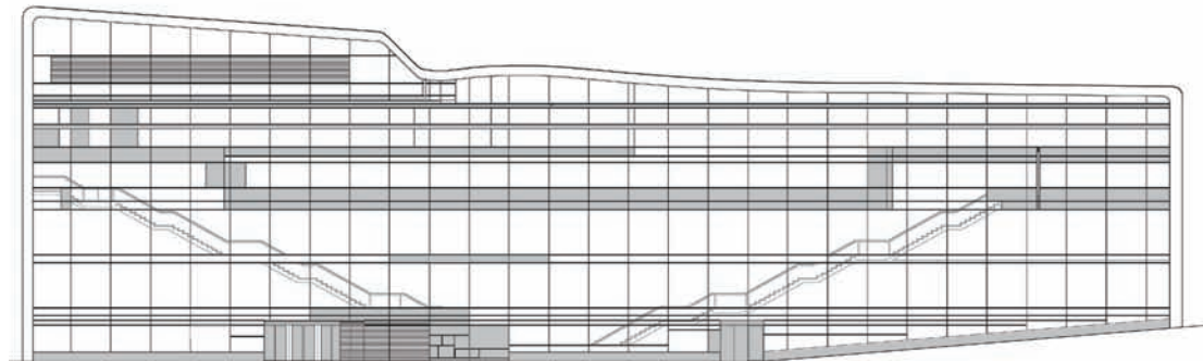
ALZADO OESTE / WEST ELEVATION
