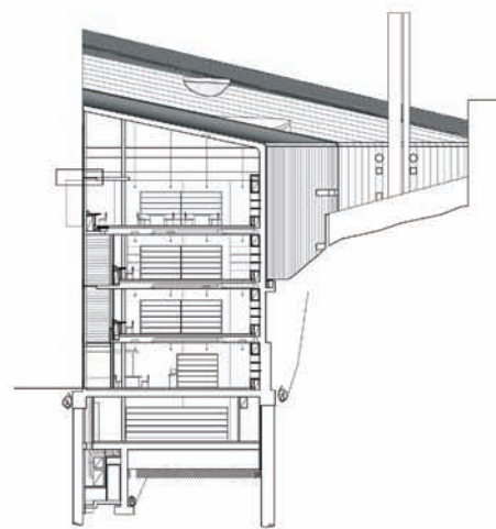
SECCION TRANSVERSAL / CROSS SECTION
