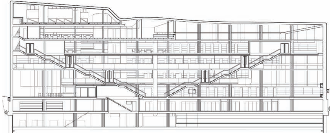
SECCION LONGITUDINAL / LONGITUDINAL SECTION
